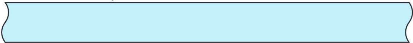
F1(A), F19(B), F23(C), F25(D) Radio Receiver Assembly
